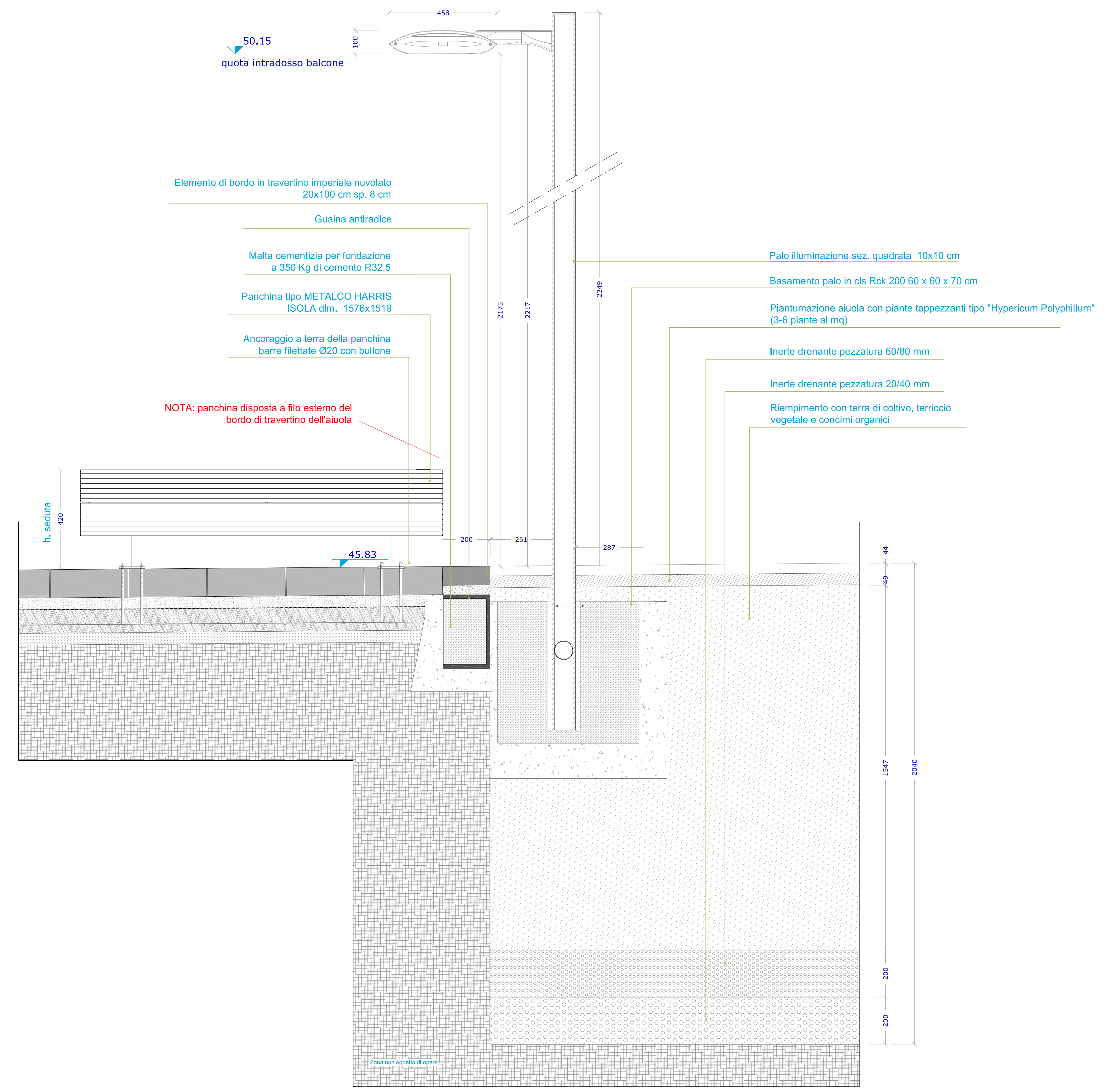
particolare 8 | scala 1:10
