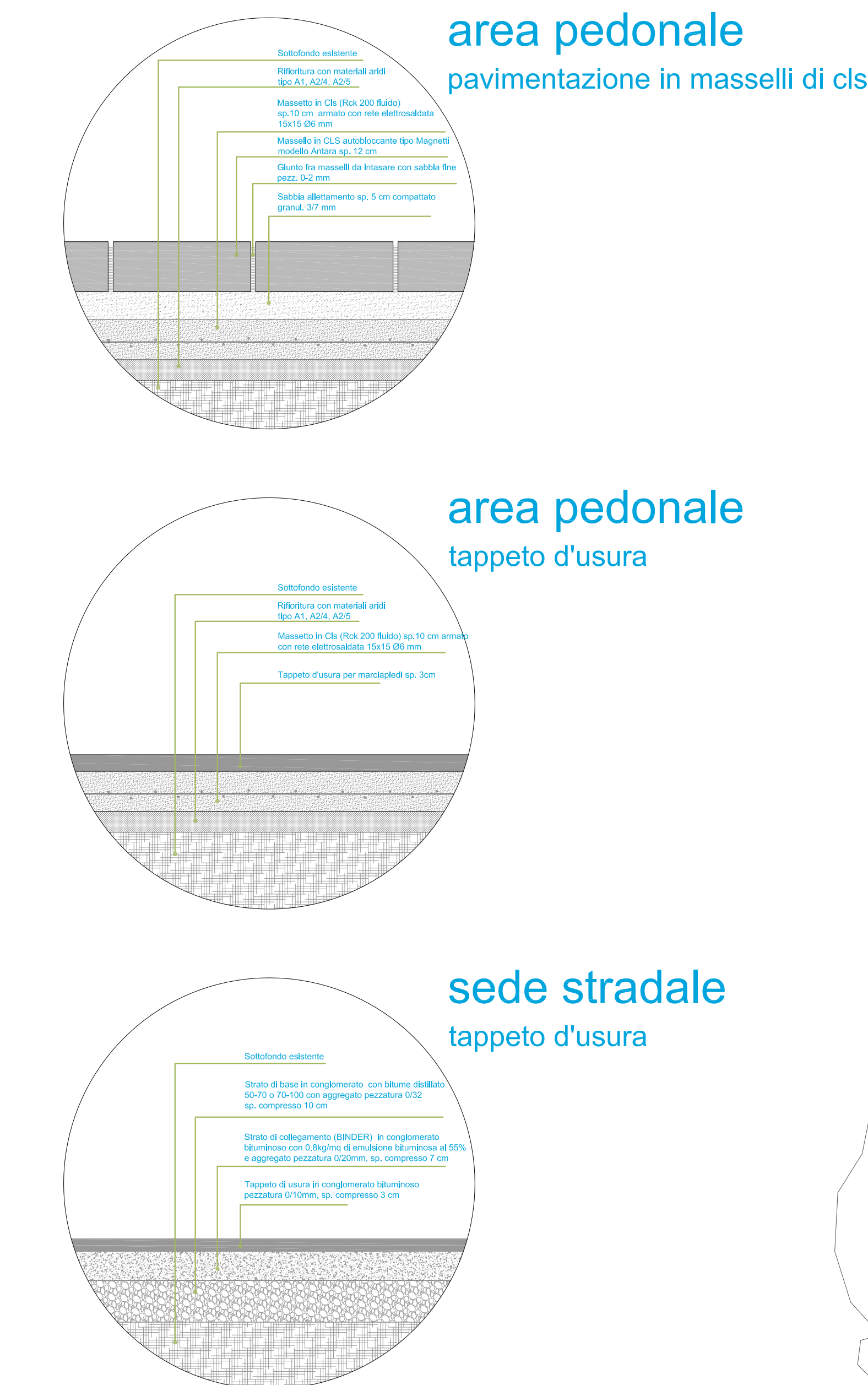
sezioni tipo | scala 1:10
