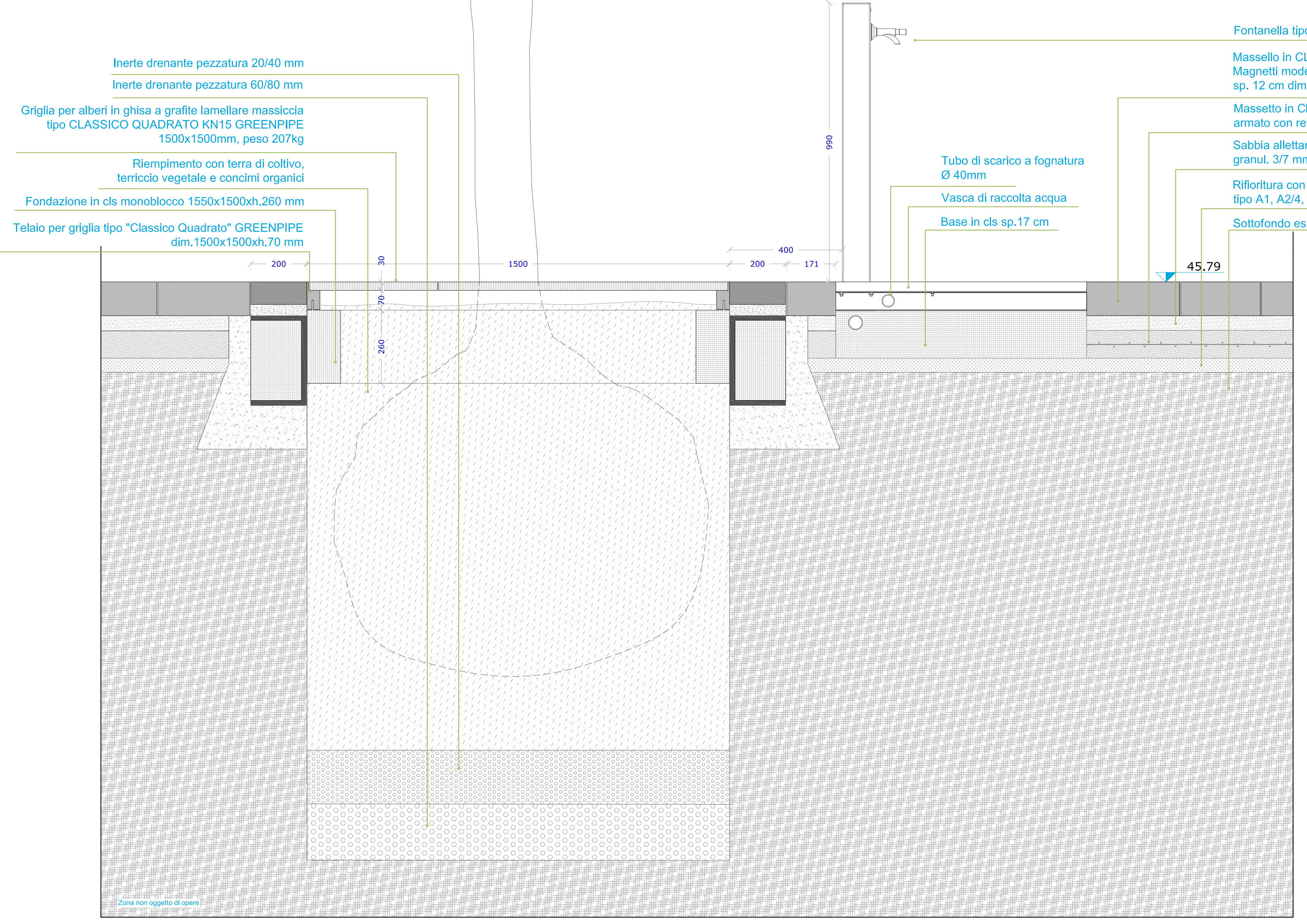
particolare 10 | scala 1:10
