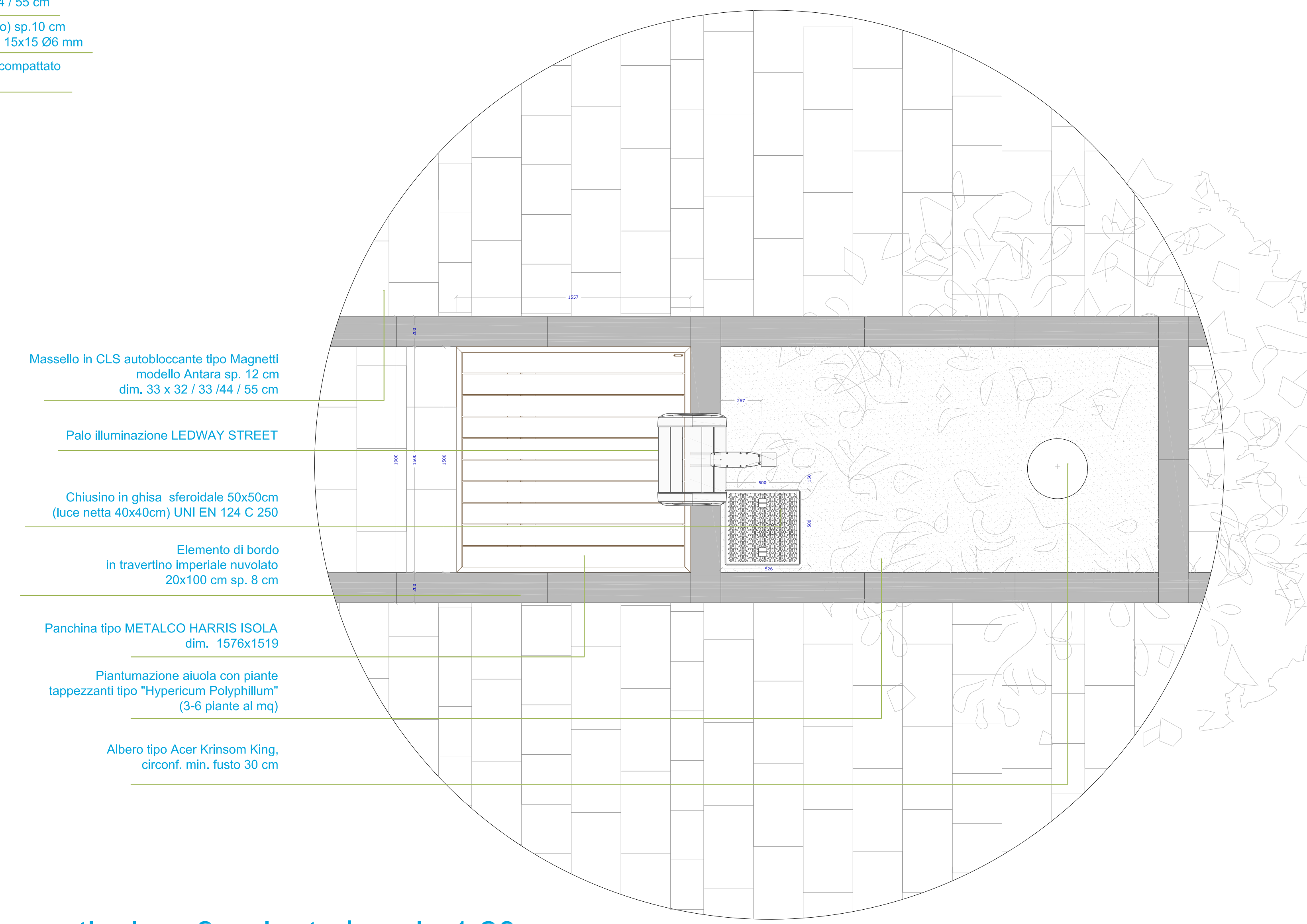
particolare 8 - pianta | scala 1:20
