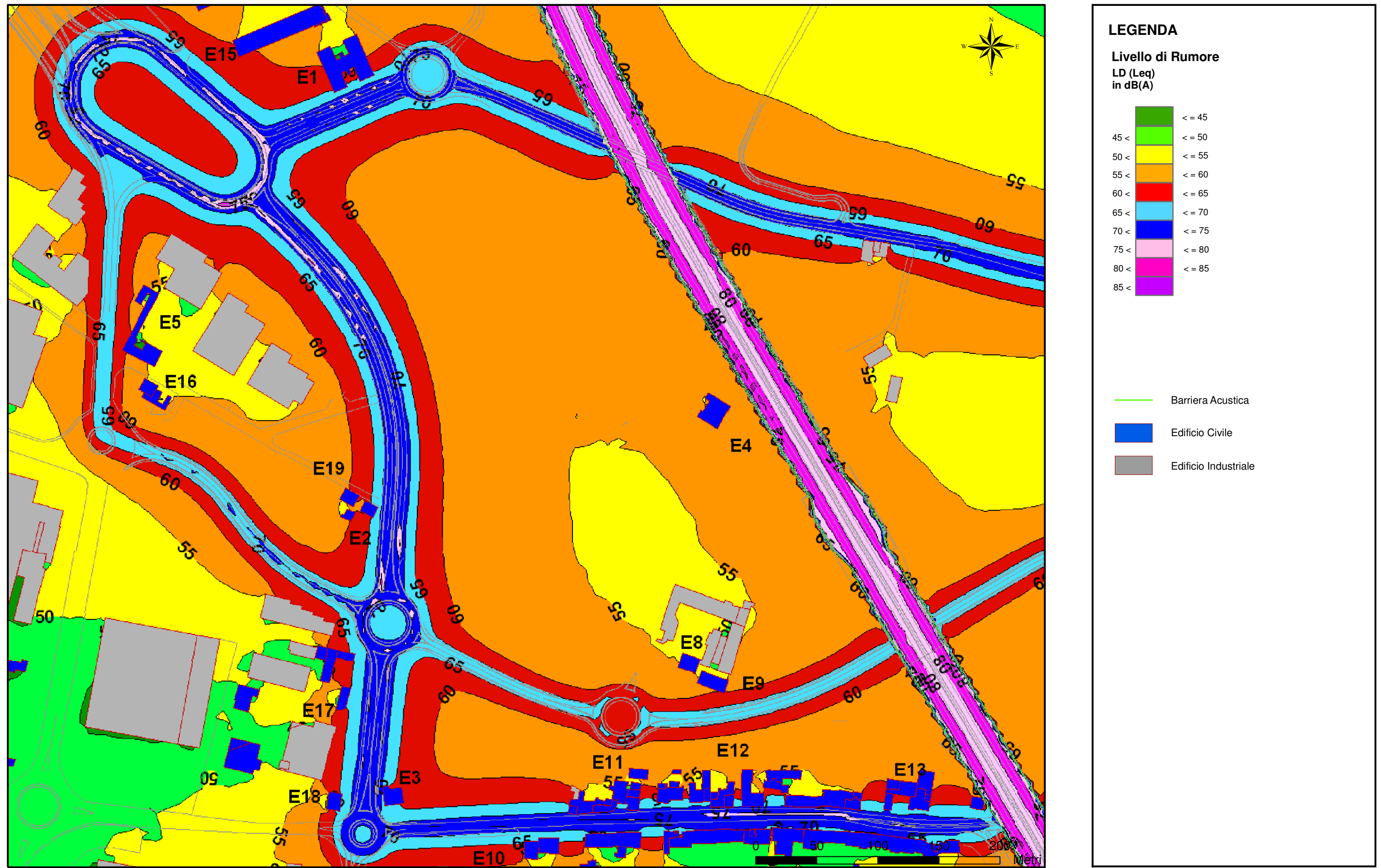
Figura 4.3.4c Ante Operam - Isofoniche Relative al Traffico per lo Scenario 4 nel Periodo Diurno
