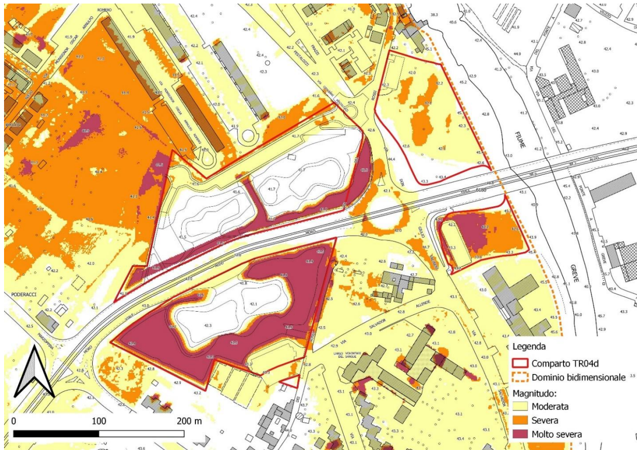
Figura 5-4 – Magnitudo idraulica ai sensi della L.R.41/2018 stato di progetto
