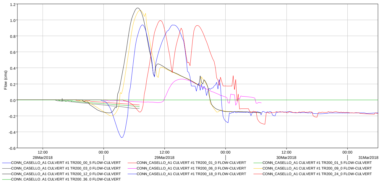
Figura 6-14 – Idrogrammi Tr 200 CONN_CASELLO_A1_C1
