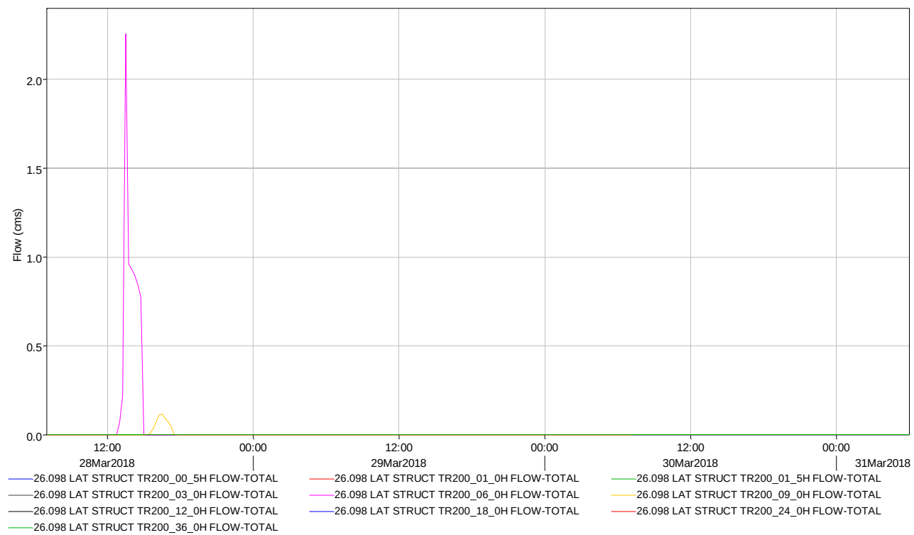
Figura 6-25 – Idrogrammi Tr 200 BC_GREVE_26.198
