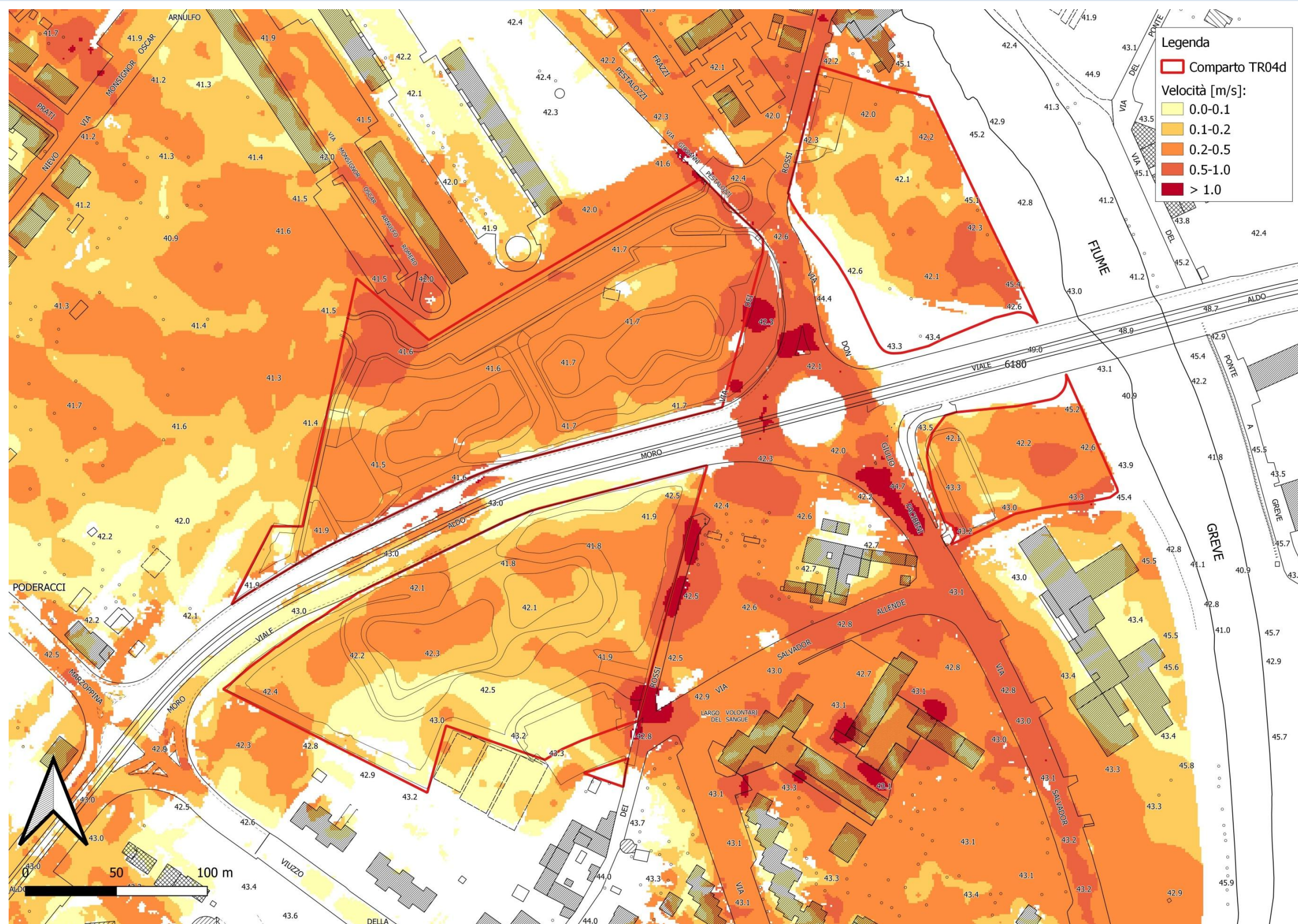
Figura 7-3 – Velocità di propagazione stato attuale Tr 200 anni
