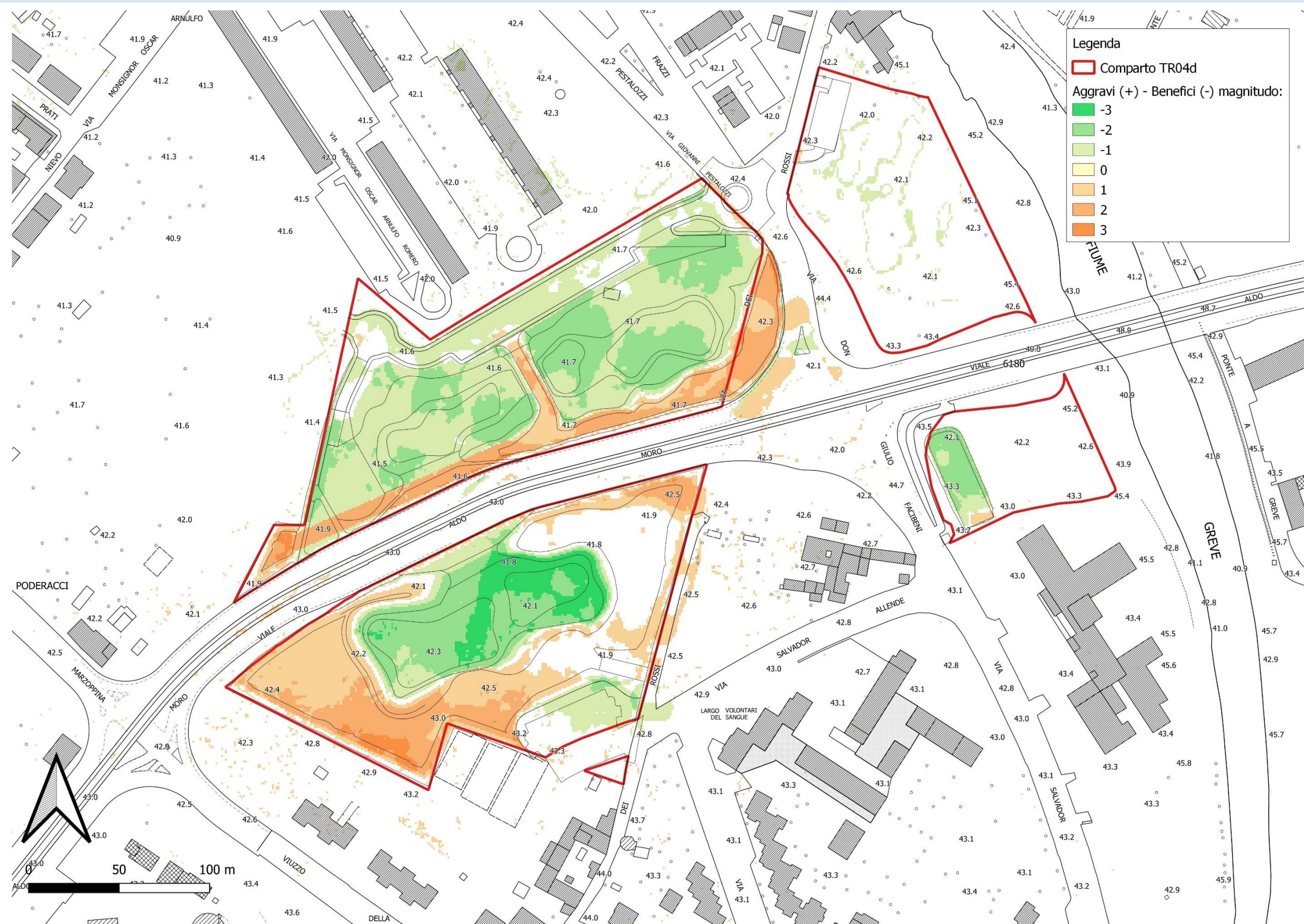
Figura 9-3 – Confronto magnitudo idraulica stato progetto – stato attuale
