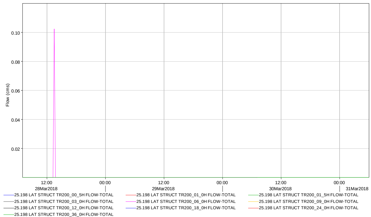
Figura 6-24 – Idrogrammi Tr 200 BC_GREVE_25.198
