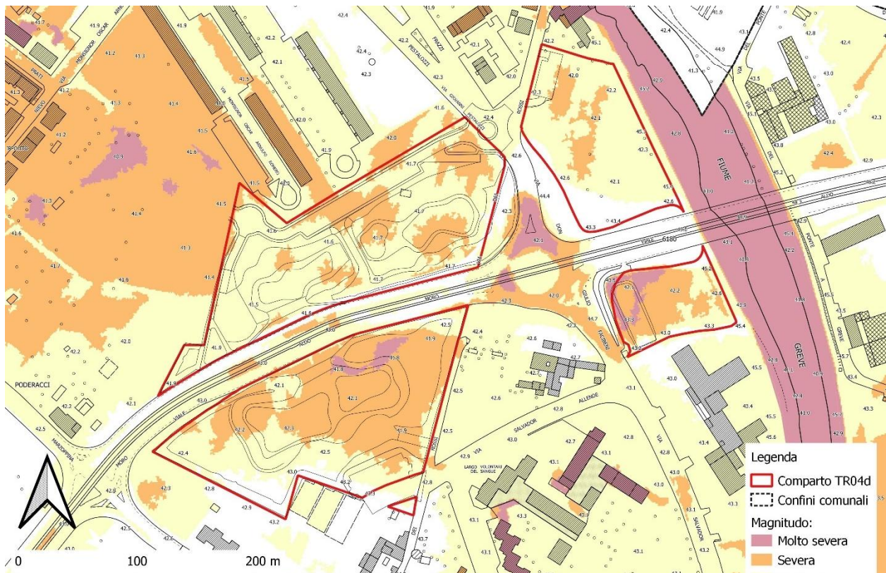
Figura 3-3 – Sovrapposizione planimetria intervento e magnitudo idraulica attuale ai sensi della L.R. 41/2018 PO Scandicci
