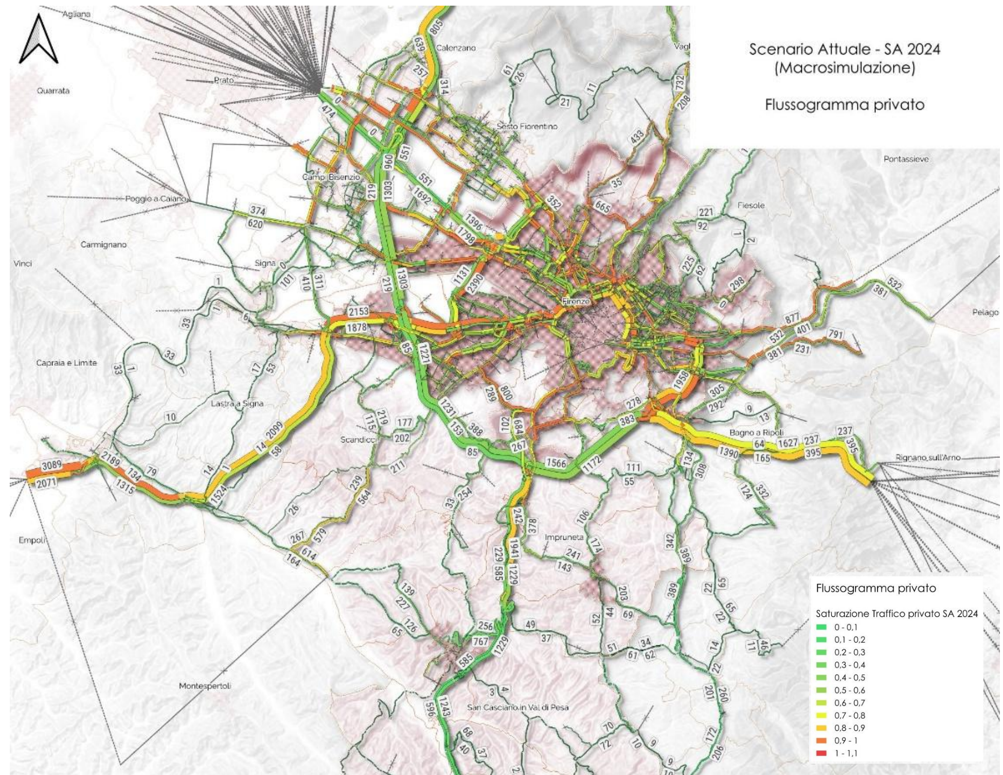
Figura 6.1 - Flussogramma di saturazione – scenario di riferimento – ora di punta mattutina
