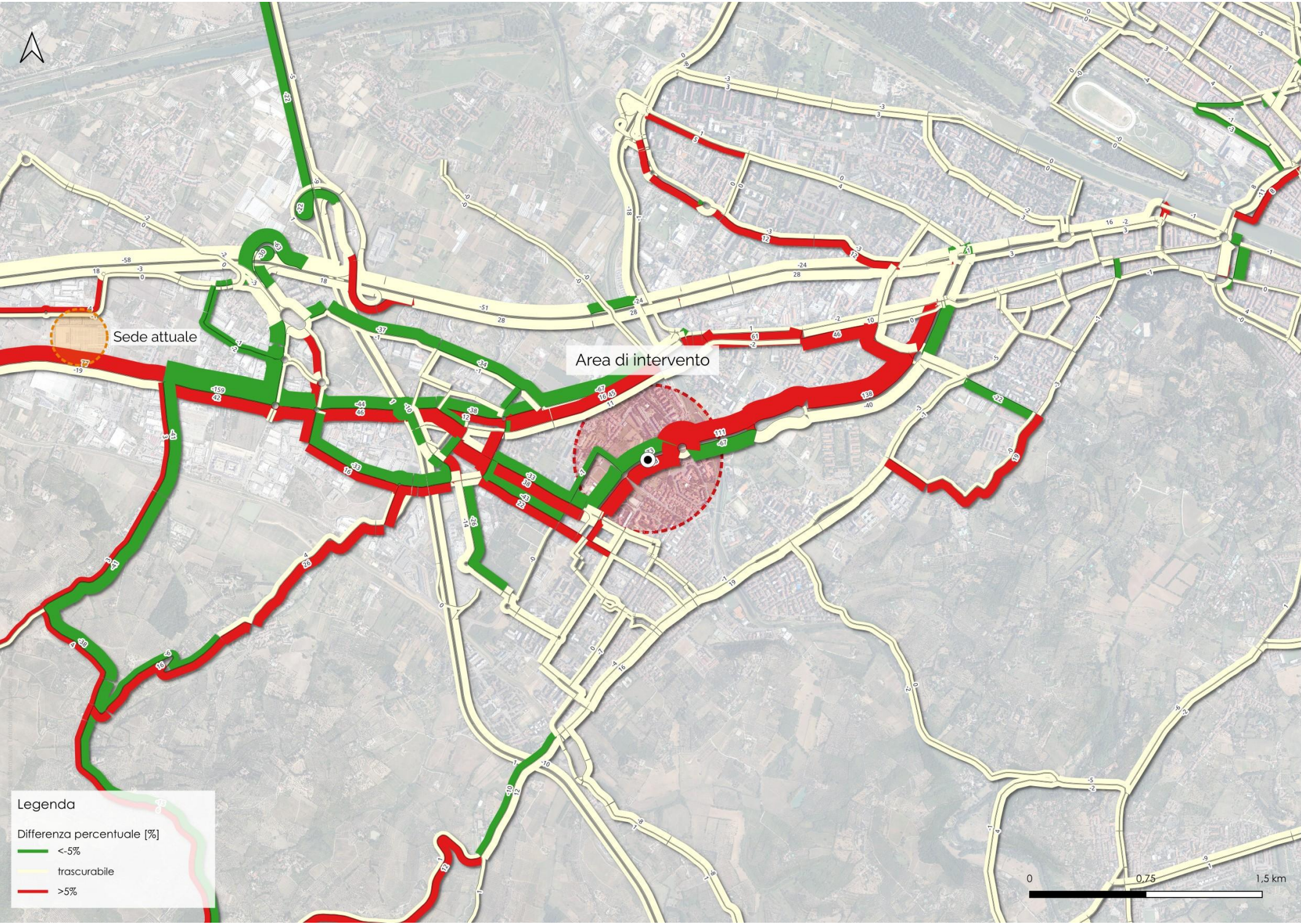
Figura 6.5 - Flussogramma differenza - percentuale di variazione dei flussi di previsione - ora di punta mattutina
