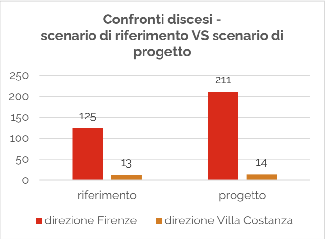
Figura 6.4 - Confronti discesi - scenario di riferimento VS scenario di progetto
