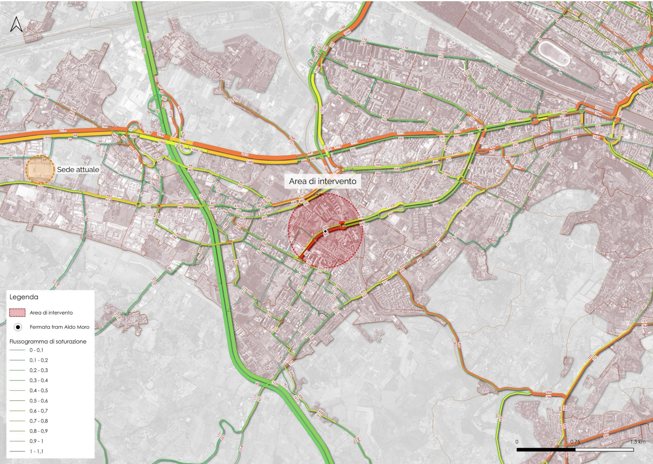
Figura 6.3 - Flussogramma di saturazione – scenario di progetto – ora di punta mattutina
