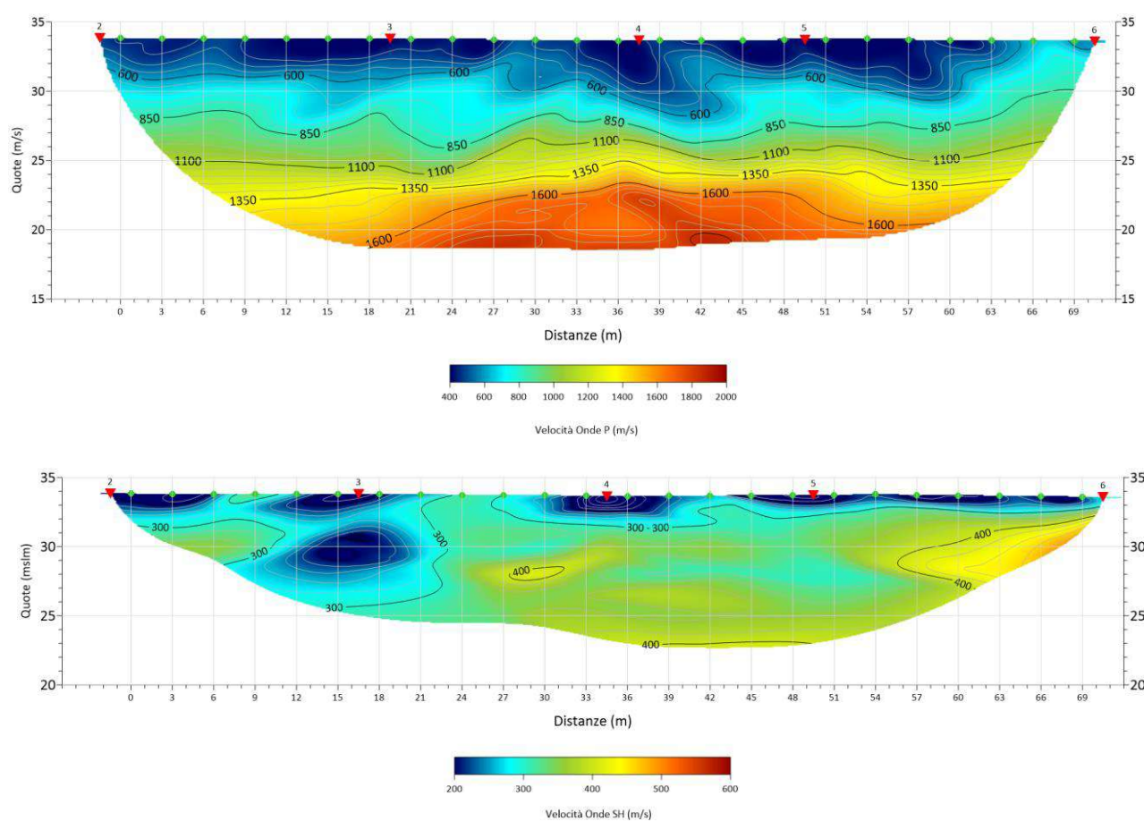
Tomografia sismica 3-3'- Onde P (sopra) ed SH (sotto).
